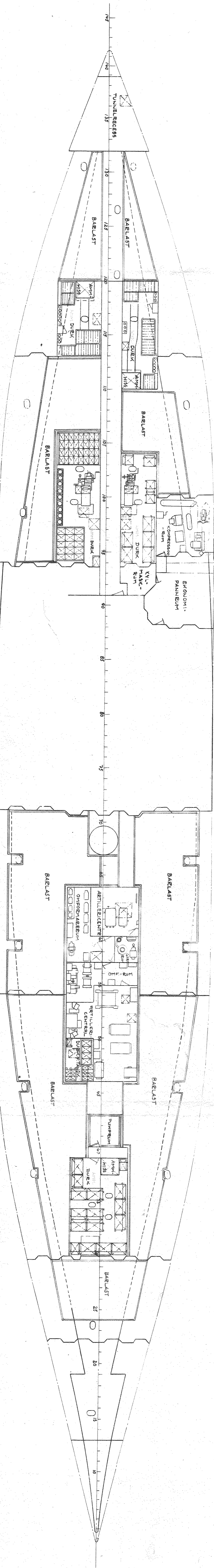
HÅLSKEPP
